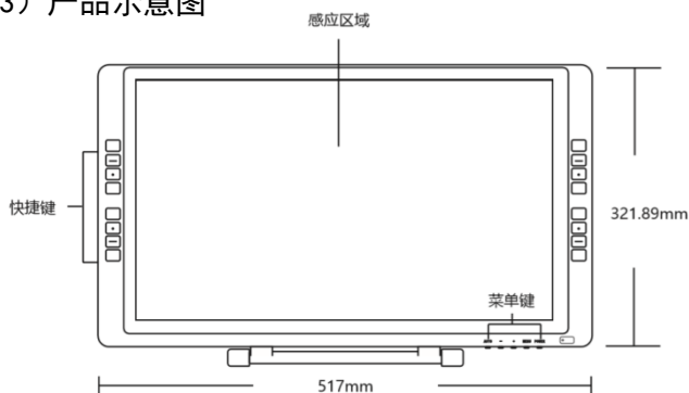
图 1-3-1.产品正面示意图
