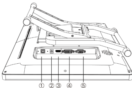
图 3-1.接口示意图
